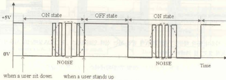
그림 6 소파 센서에서의 잠음 신호 보정
