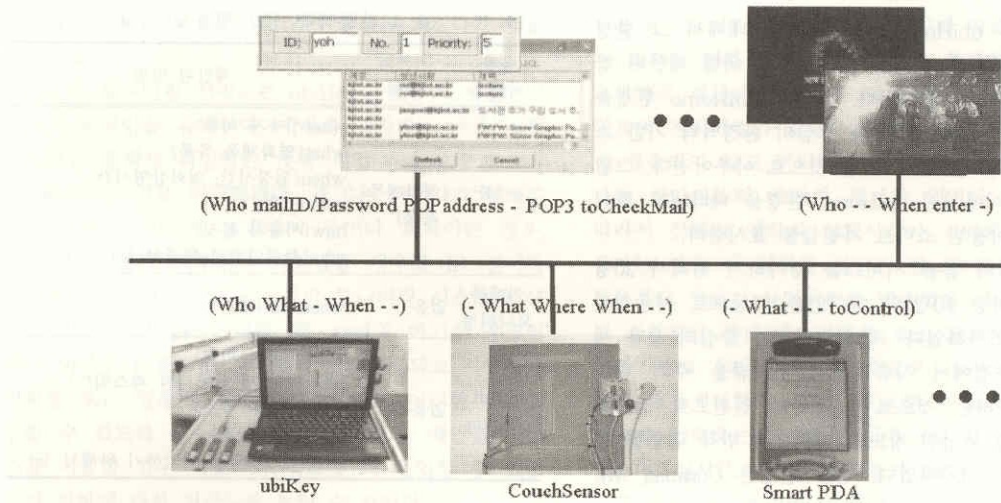
그림 14 제안된 cMail checker와 각 센서와의 연결도
