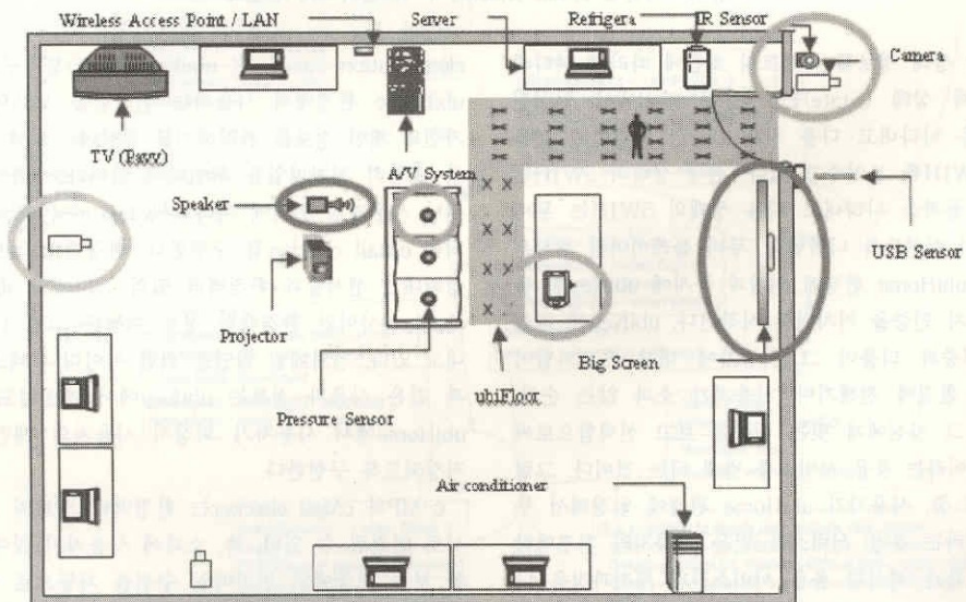
그림 15 ubiHome 테스트 베드
