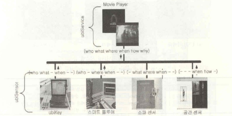
그림 11 제안된 c-MP와 사용된 센서들과의 연결도
