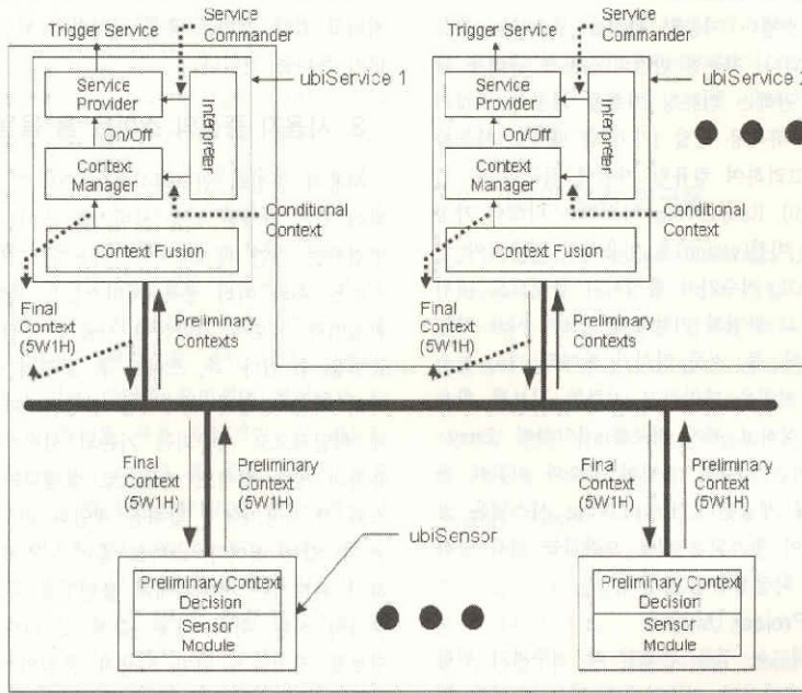
그림 1 ubi-UCAM을 이용한 응용 서비스 모형의 구조
