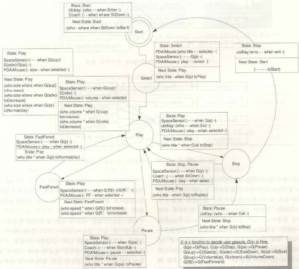
그림 12 c-MP의 상태 정보 및 환경대략 조건 정보
